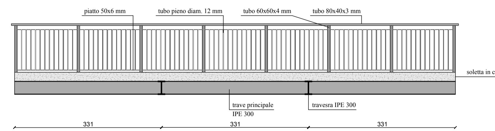
PROSPETTO - scala 1:50
