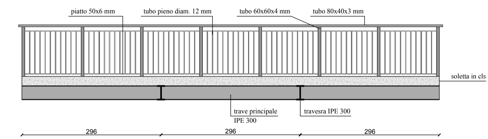
SEZIONE 2-2 - scala 1:50
