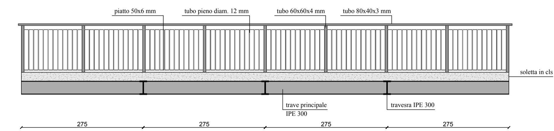
PROSPETTO - scala 1:50
