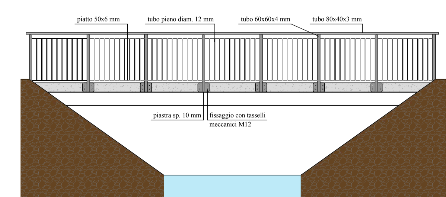
SEZIONE 1-1 - scala 1:20
