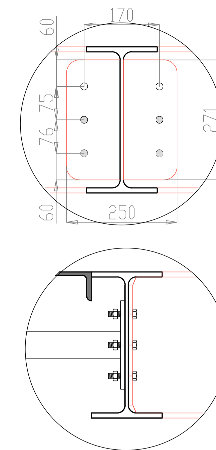
DETTAGLIO SEZIONE B-B Scala 1:5
