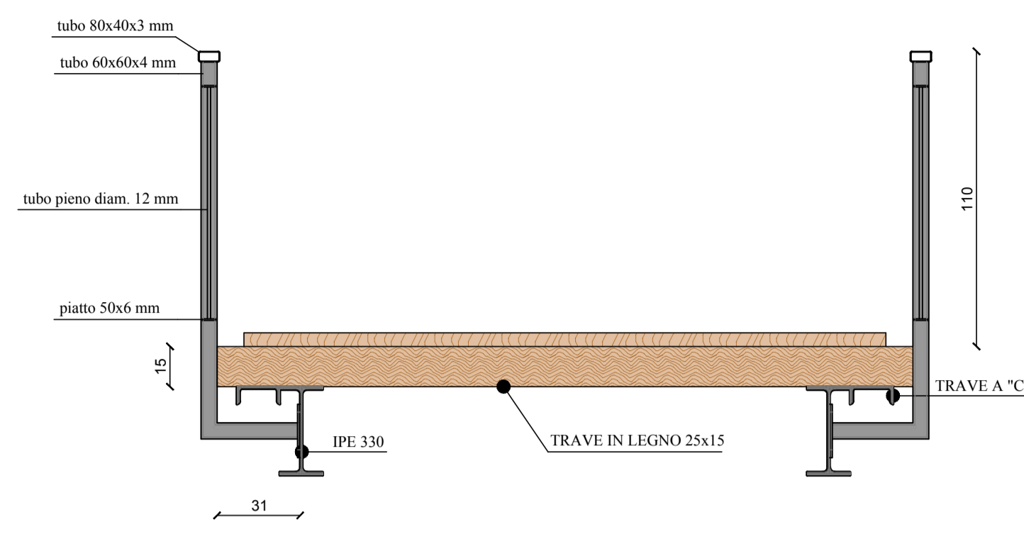
SEZIONE 1-1 - scala 1:20
