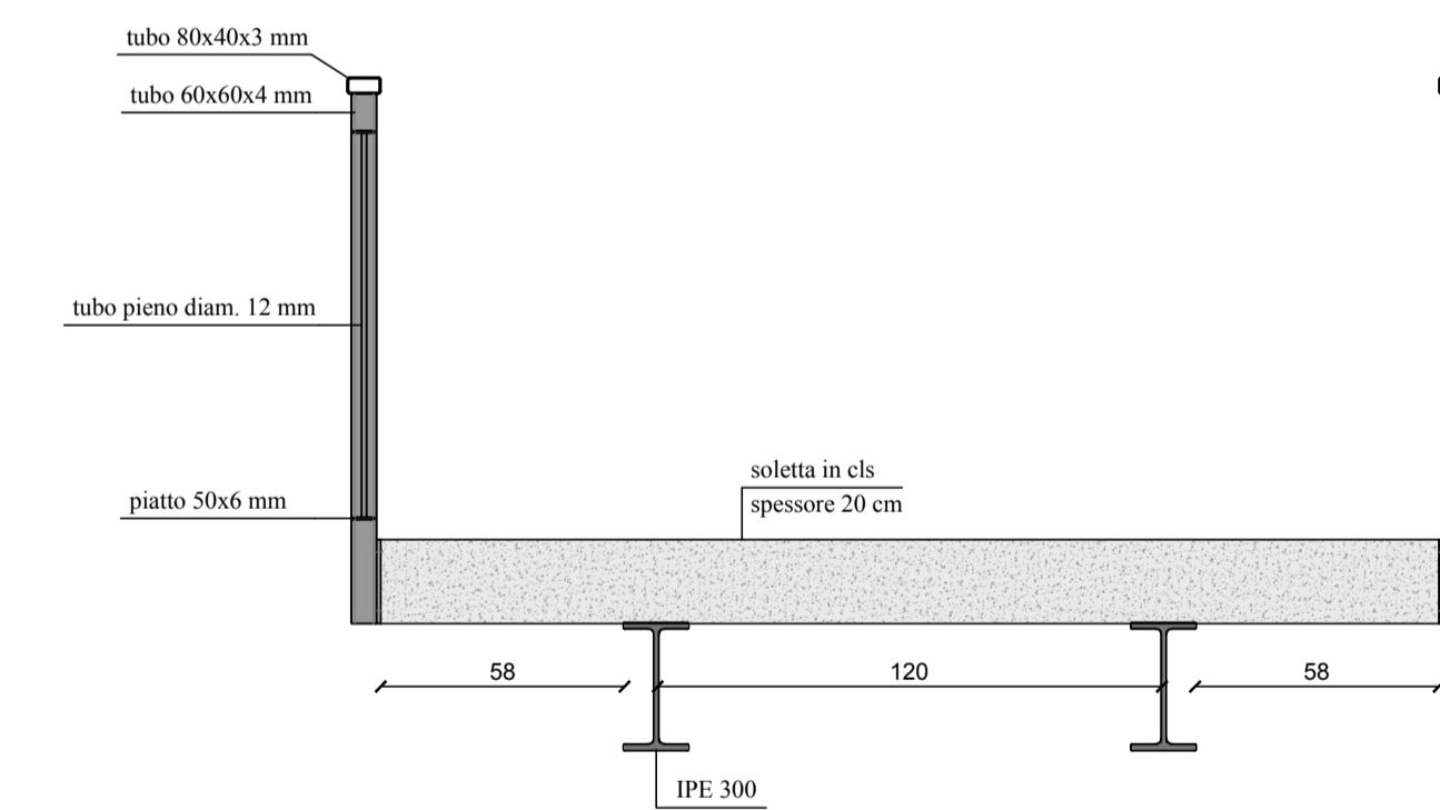
SEZIONE 2-2 - scala 1:50
