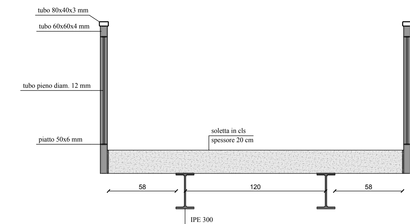
SEZIONE 2-2 - scala 1:50
