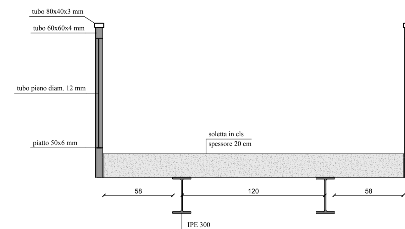
SEZIONE 2-2 - scala 1:50
