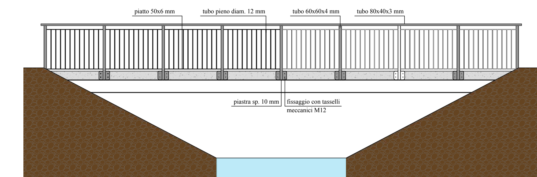
PROSPETTO - scala 1:50
