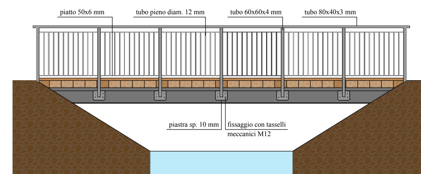
PROSPETTO - scala 1:50
