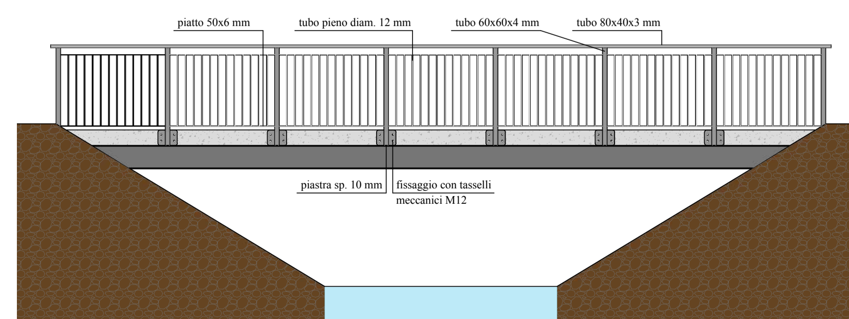
PROSPETTO - scala 1:50
